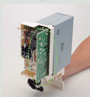
Des étapes simples pour retirer la carte électronique
