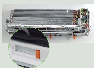
Fixation par clip pour un retrait facile de la grille de refoulement
